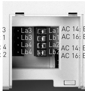
Abb. 6: Geöffnetes Anschlussfeld
